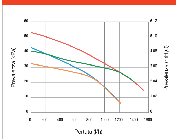
Grafico portata e prevalenza
